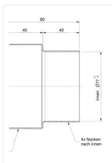
Dessin coté
