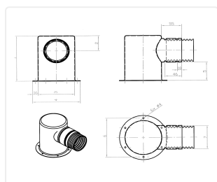
Dessin coté
