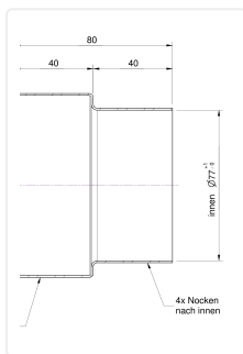
Masszeichnung
