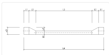
Masszeichnung
